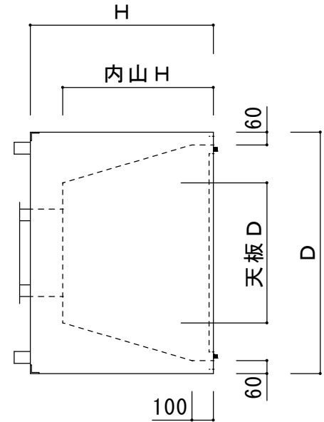
油受け W溝詳細
