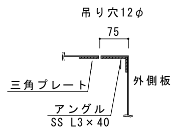
吊り詳細
